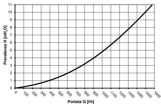
Grafico perdite di carico modulo idraulico lato pompa di calore
