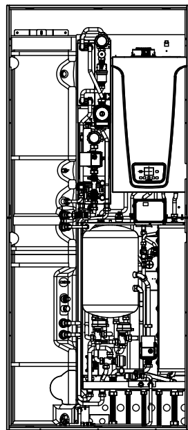
CSI IN Auriga H WI-FI con modulo solare (fornito come accessorio)
