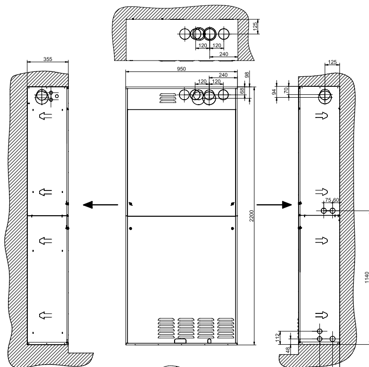
CSI IN Auriga H WI-FI con modulo solare (fornito come accessorio)
